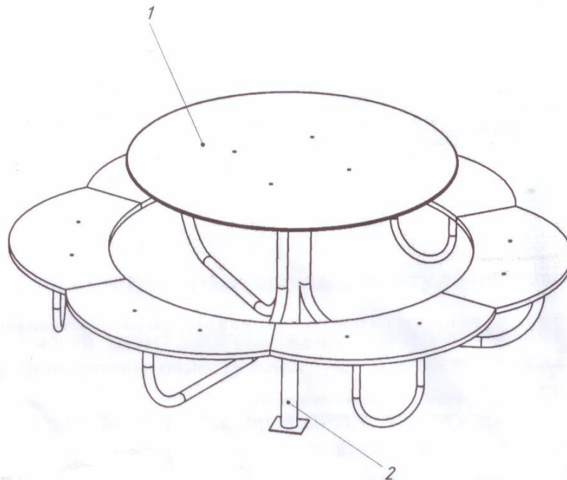
Рисунок 2- схема сборки
